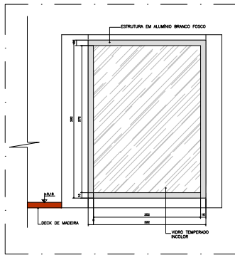
VISTA 02 ESC 1/20
