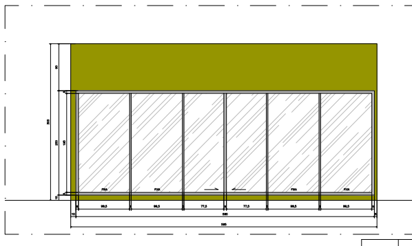
VISTA 03 ESC 1/20
