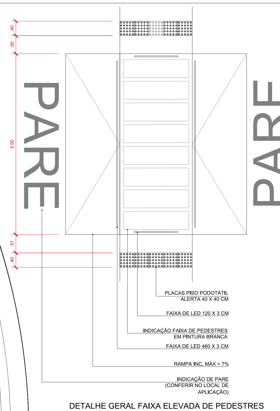
DETALHE GERAL FAIXA ELEVADA DE PEDESTRES ESCALA 1:50
